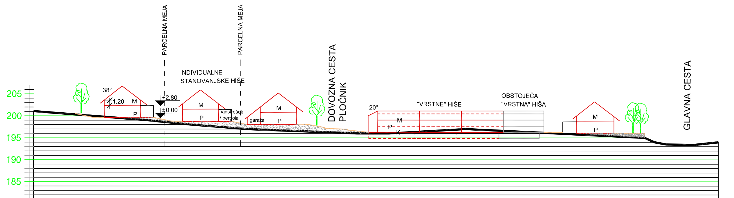
PREREZ B-B
