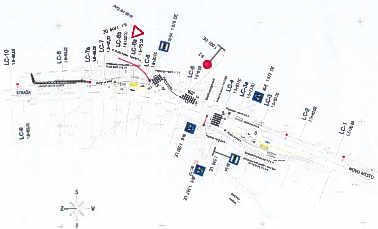
Slika 2: Izvedbeni načrt za izvedbo – prometna situacija
